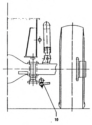
Schnitt A - B
